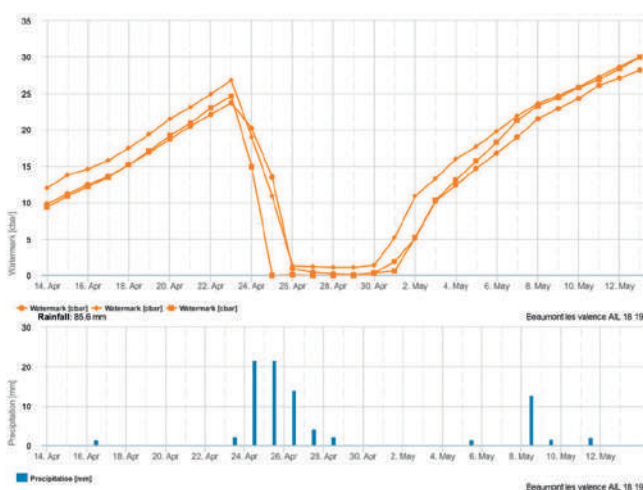
Valeurs enregistrées par la station météo et les sondes Watermark du 14 avril au 12 mai, Beaumont les Valence - Source : CA26
